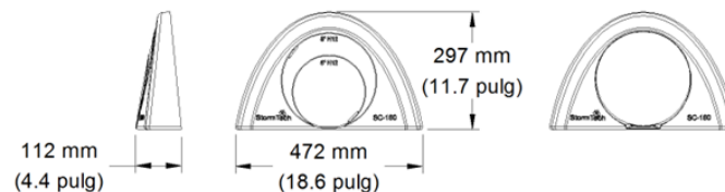
Figura 4. Dimensiones de la tapa SC-160LP y guías de corte para insertar tubos de entrada o salida
