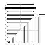
Codo con empaque campana - espiga
