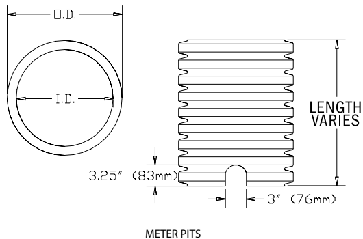
METER PITS
