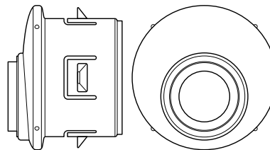
Reductor a tubo de PVC
