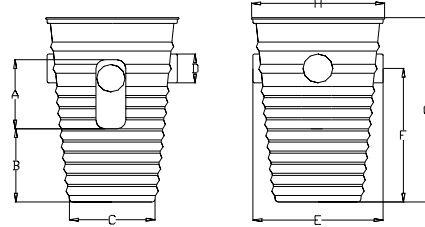
Sumidero y tapa del eyector
